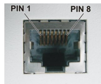
Fig. 4.10: RJ-45F
