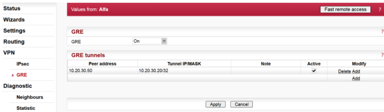
Fig. 7.8: Menu GRE
